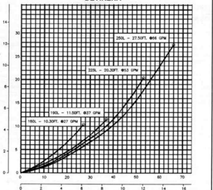
CURVA DE CAIDA DE PRESIÓN DOMÉSTICA DE FILTROS DE ARENA
